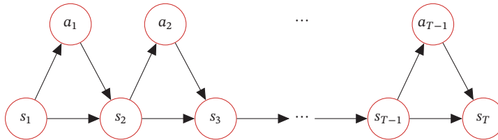
图 14.3 马尔可夫决策过程
