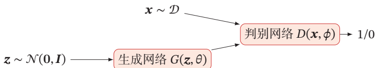
图 13.8 生成对抗网络的流程图
