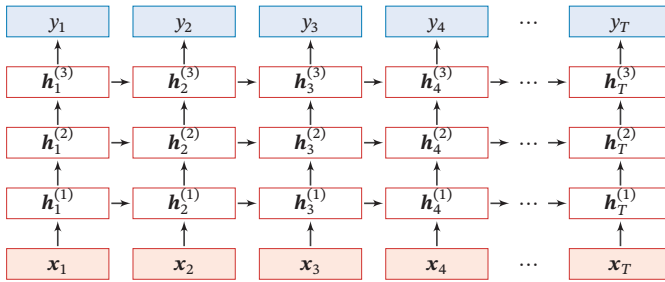
图 6.9 按时间展开的堆叠神经网络
