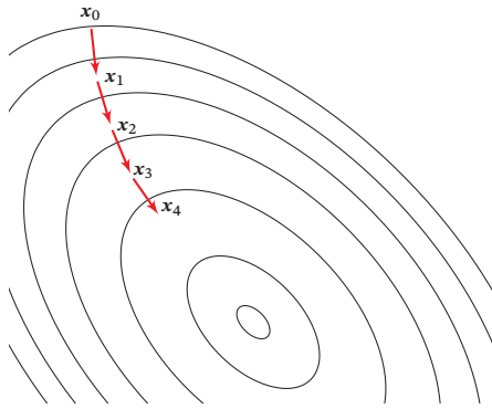
图 C.1 梯度下降法
