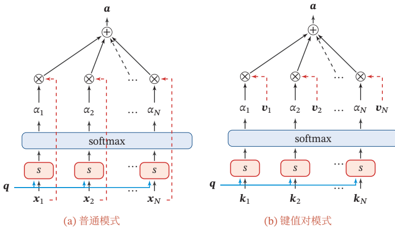
图 8.1 注意力机制
