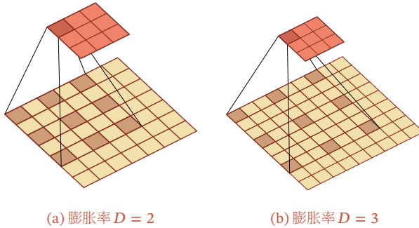
图 5.18 空洞卷积
