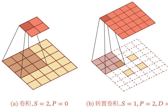
图 5.17 步长 S = 2 , 无零填充 P = 0 的二维卷积和其对应的转置卷积
