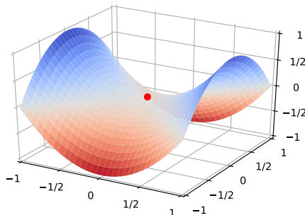
图 7.1 鞍点示例
