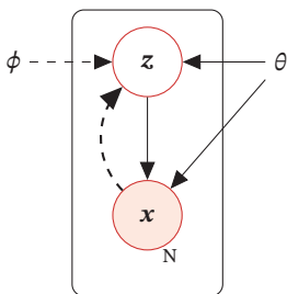
图 13.3 变分自编码器
