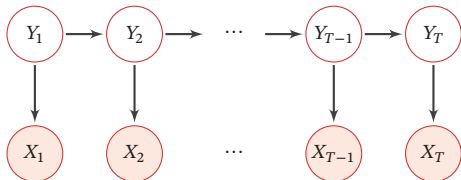
图 11.6 隐马尔可夫模型
