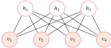
图 12.3 一个有 7 个变量的受限玻尔兹曼机
